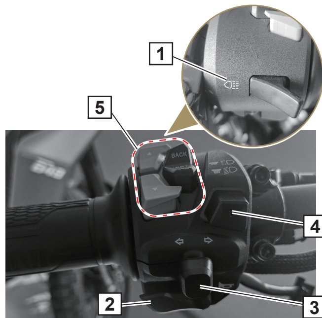
Interruptor manubrio izquierdo
